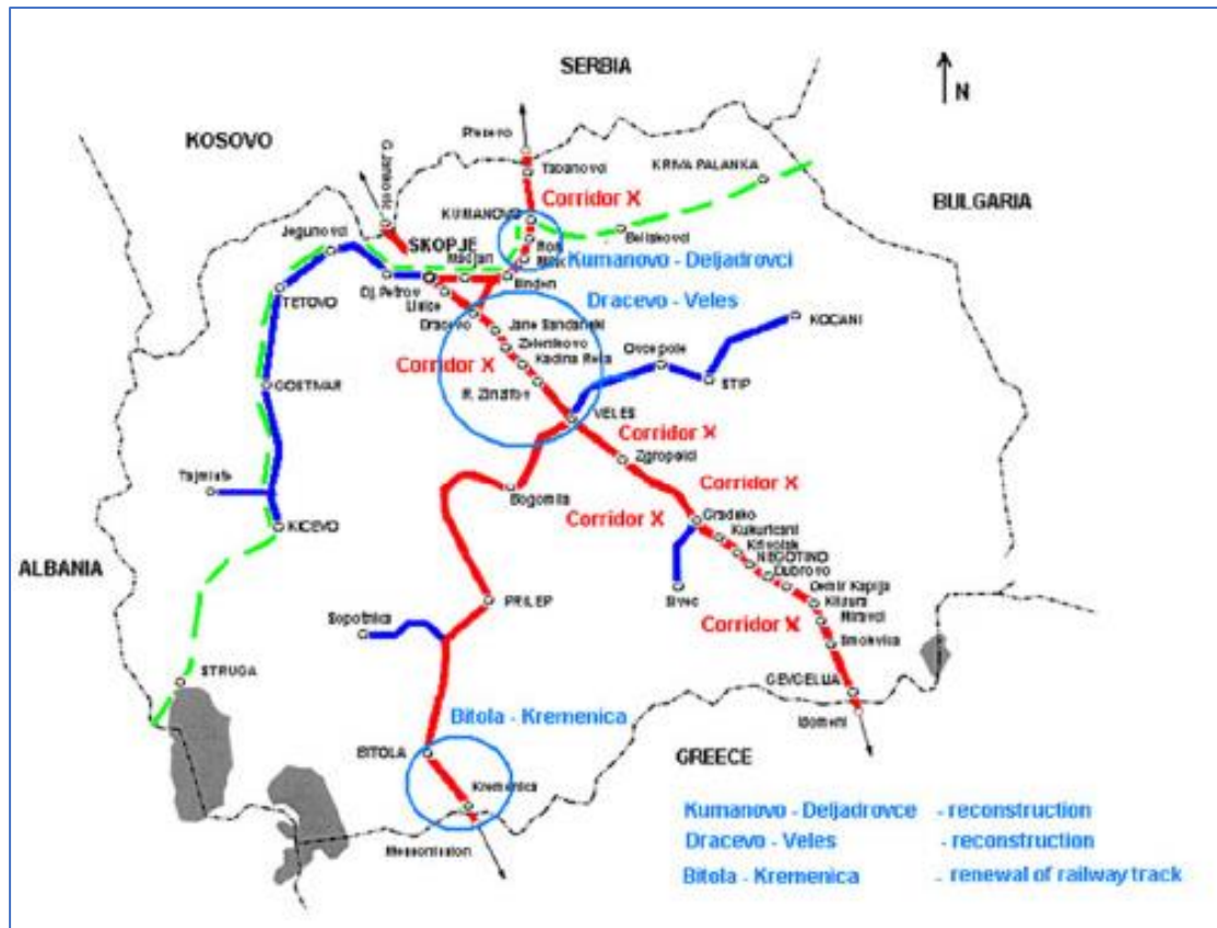
Εικόνα 3: Σιδηροδρομικό δίκτυο, υπό αναβάθμιση δίκτυο διαδρόμου Χd Πηγή: ADT Omega http://www.adtomega.gr/portfolio2.php?page=port2&id=37&lang=2
